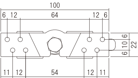
Rol Pintu Gantung Tugas Berat
