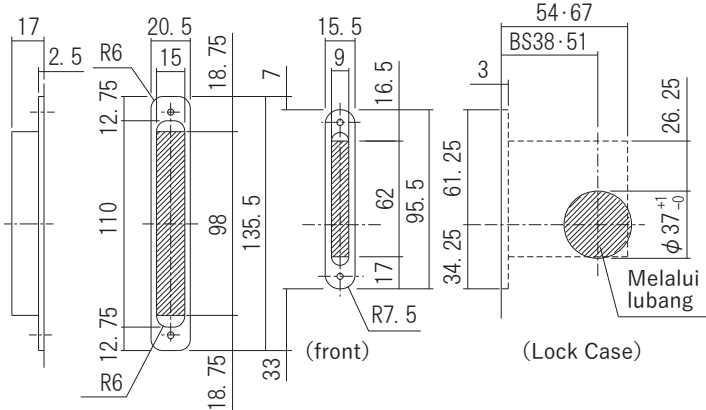
Desain penggalan Strike Desain penggalan Lock Case
