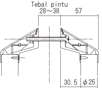
Potongan A-A
